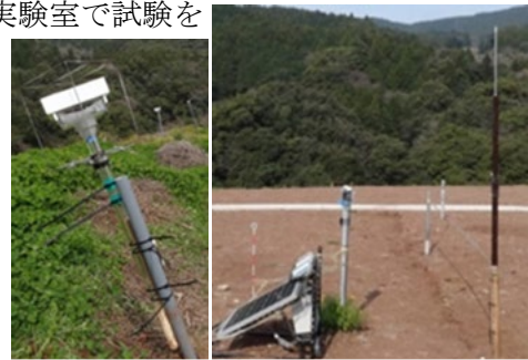
ケージ及び簡易避雷針のフィールドテスト
