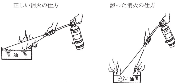
図 1.3 油火災の消火方法
